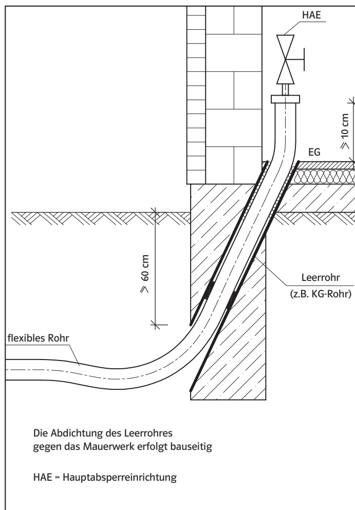
nicht unterkellerte Gebäude
