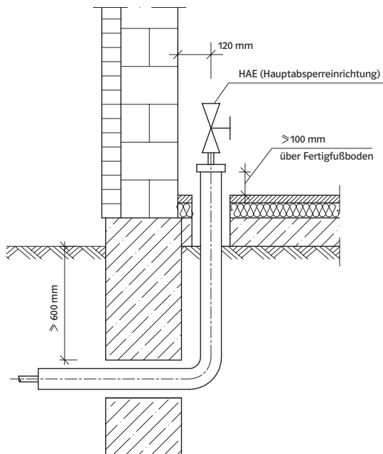
Schnitt A-A
