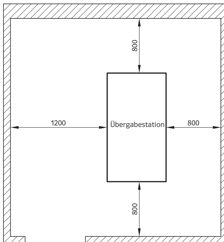
Freistehende Übergabestationen
