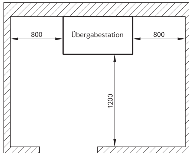
Wandhängende und auf Grundrahmen montierte Übergabestationen
