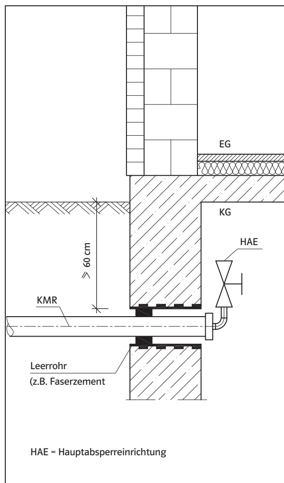
unterkellerte Gebäude
