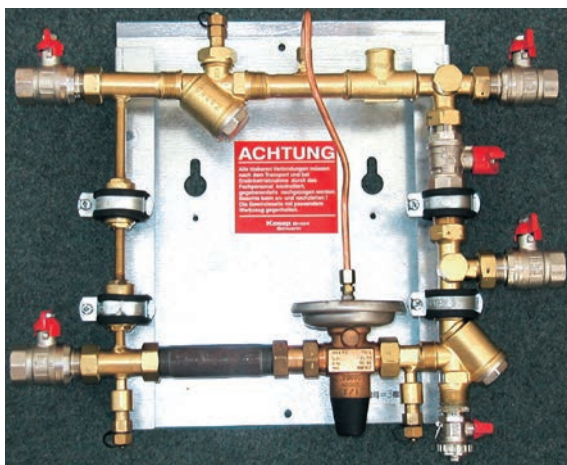
Basis-D Universalstation (< 30 kW), Übergabestation direkt
